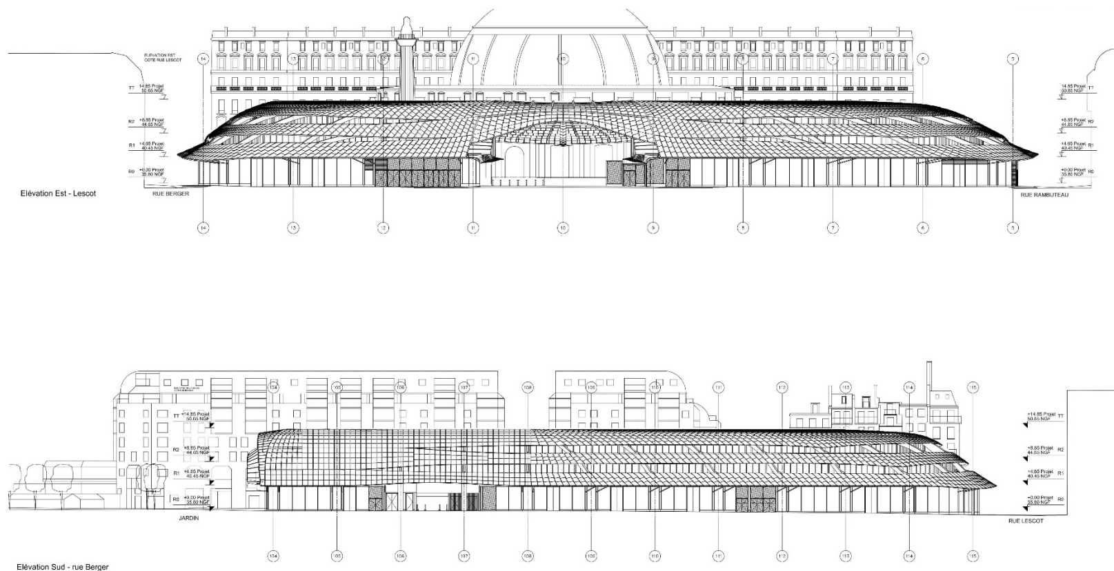
Elévations Est et Sud
