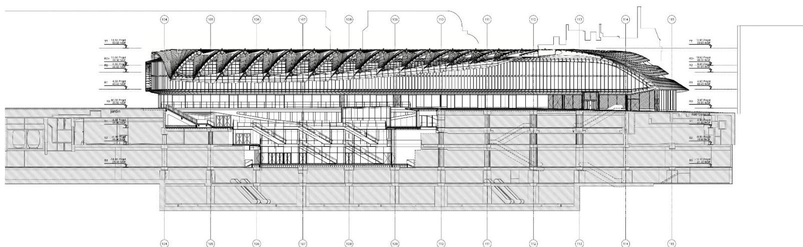
Coupe longitudinale Est-Ouest
