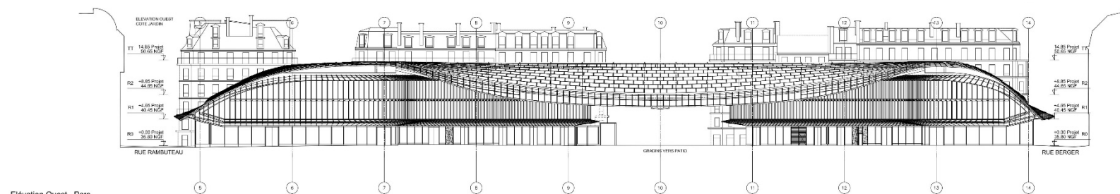
Elévation Ouest - Parc
