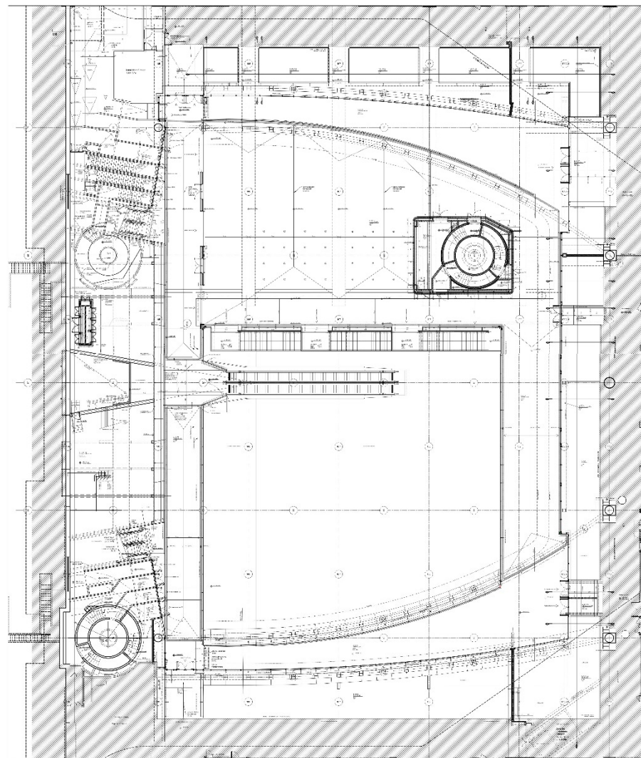
Plan du premier sous-sol
