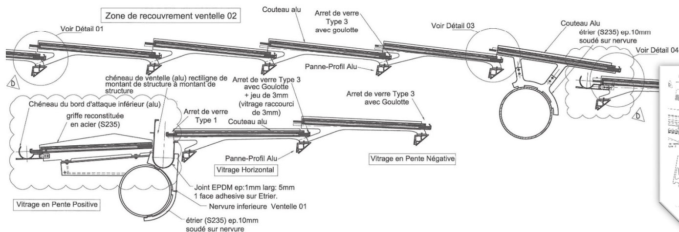
PRINCIPE SUR PENTE INVERSEE
